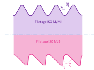
Figure 1- Comparaison profil filetage M et MJB
